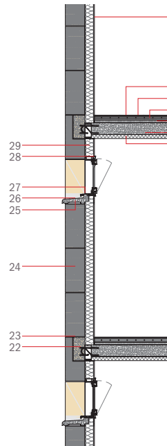
Sezione CC
