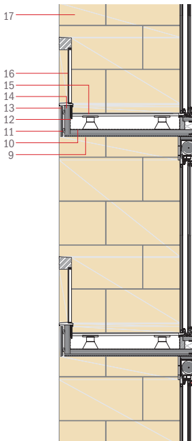
Sezione AA
