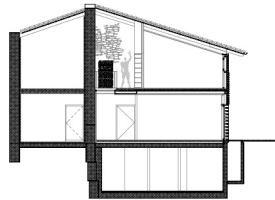
Sezione trasversale della sala multiuso
