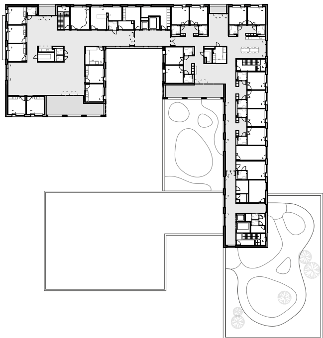
Pianta terzo piano
