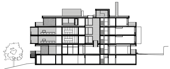
Sezione trasversale
