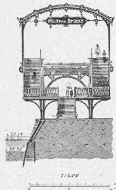
Fig. 6. Trage-Gerüst. Querschnitt.
