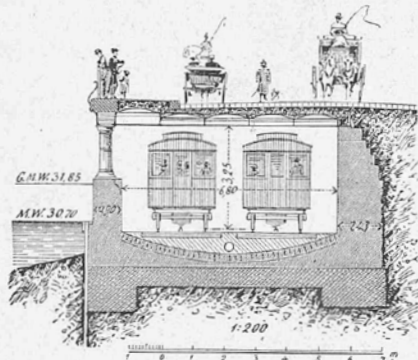
Fig. 2. Unterpflasterbahn am Reichstag-Ufer.
