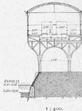
Fig. 3. Querschnitt durch den Bahnhof vor der Stütze.
