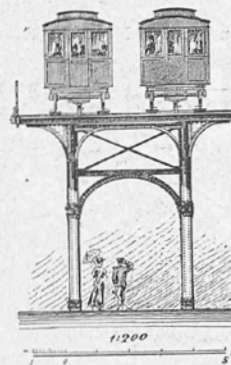
Fig. 6. Trage-Gerüst. Querschnitt.
