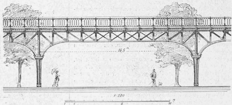
Fig. 7. Trage-Gerüst. — Ansicht.
