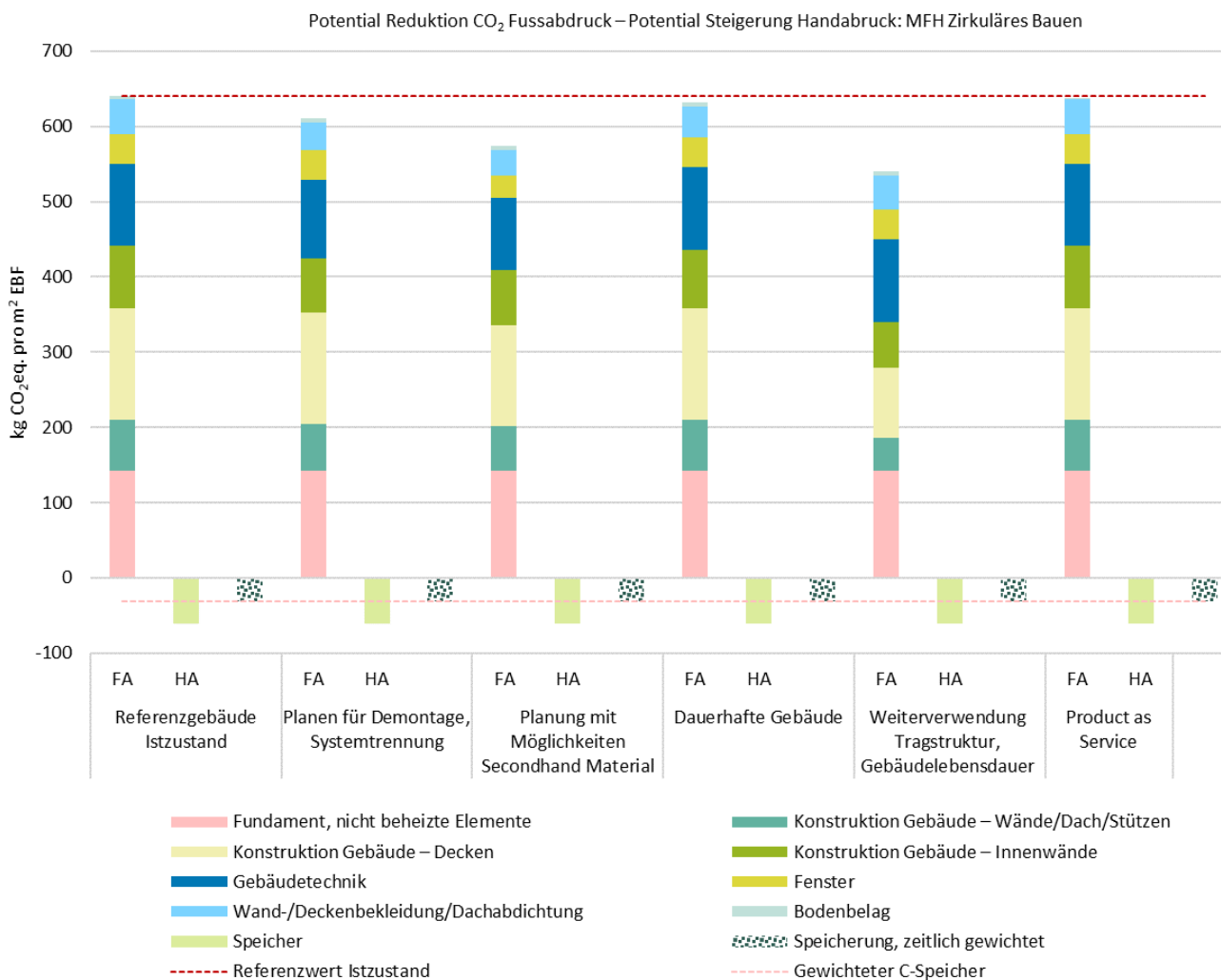
Abb. 34: Ergebnis Reduktionspotenzial der Massnahmen, hergeleitet mit einer Analyse im Vergleich zum Referenzwert Istzustand (Links; rot gestrichelte Linie). Die Wiederverwendung von Materialien und Tragstrukturen führt zu einer relevanten Reduktion des Fussabdrucks (FA). Der Handabdruck (HA) bleibt bei diesen Massnahmen unverändert. Eigene Berechnung/Darstellung.
