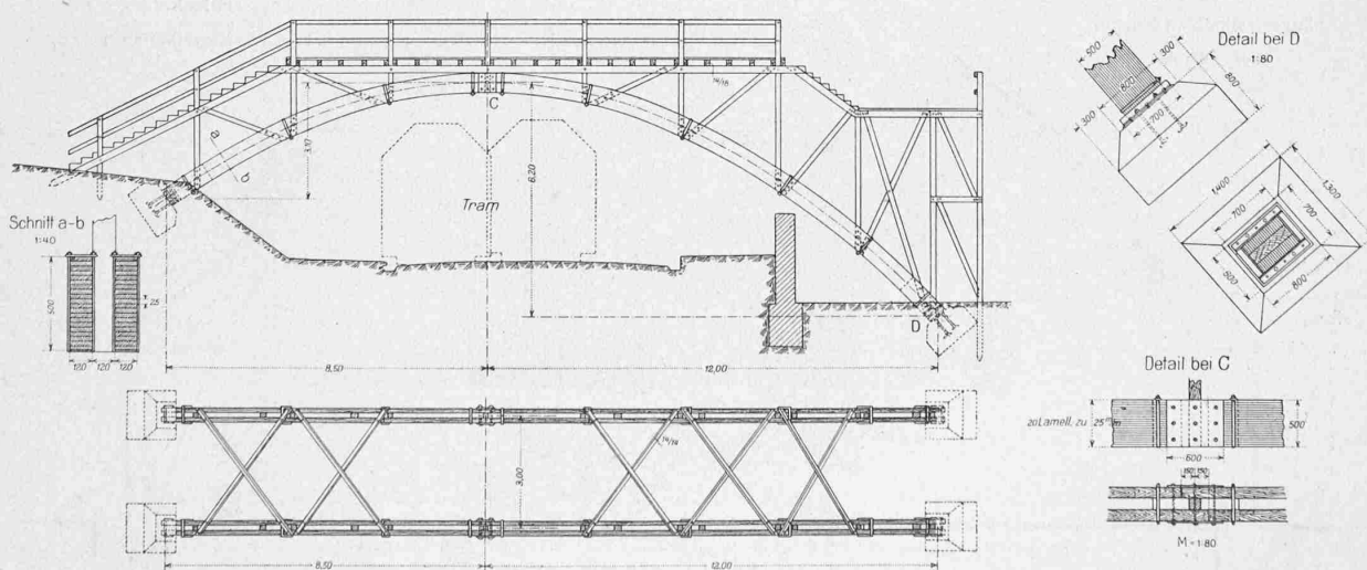
Abb. 1. Prov. Fussgängersteg bei Lausanne für 350 kg/m 2 Nutzlast. — Masstäbe 1:200, 1:80 und 1:40.
