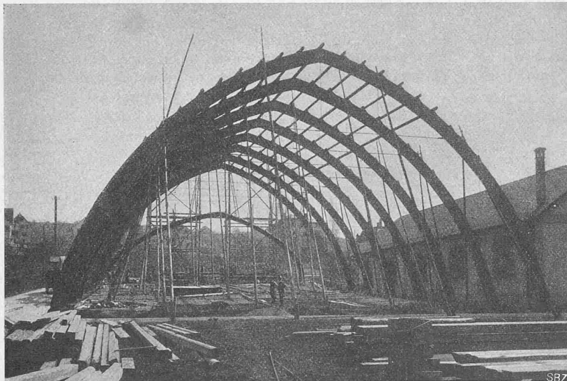
Abb. 5. Sängerställe Küssnacht bei Zürich 1911. — Stützweite 30 m.
