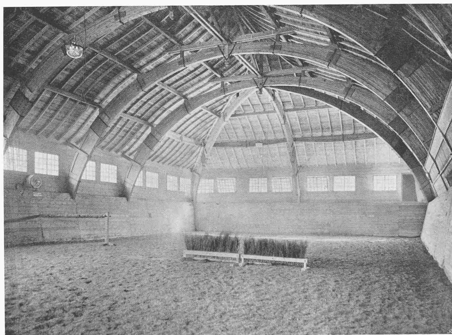
Hetz-Konstruktion von TERNER & CHOPARD, Ingenieur-Bureau Zürich
