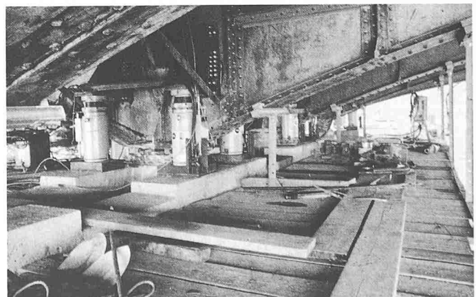
Bild 12. Aufpressen der alten Brücke unter Verkehr zum Einbau der Gleitschuhe für den Verschiebungsvorgang um etwa 1 cm
