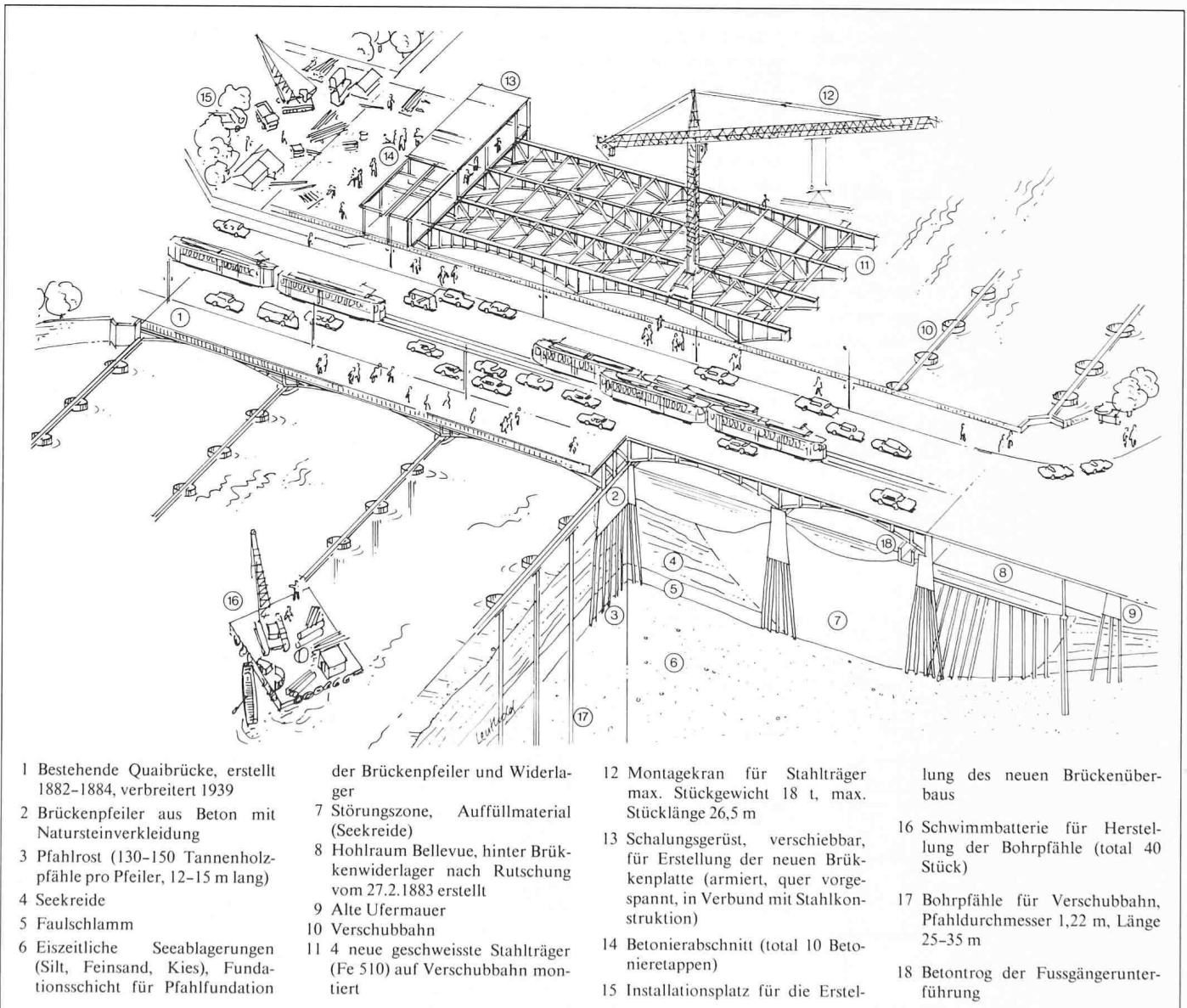
Bild 9. Bauvorgang
