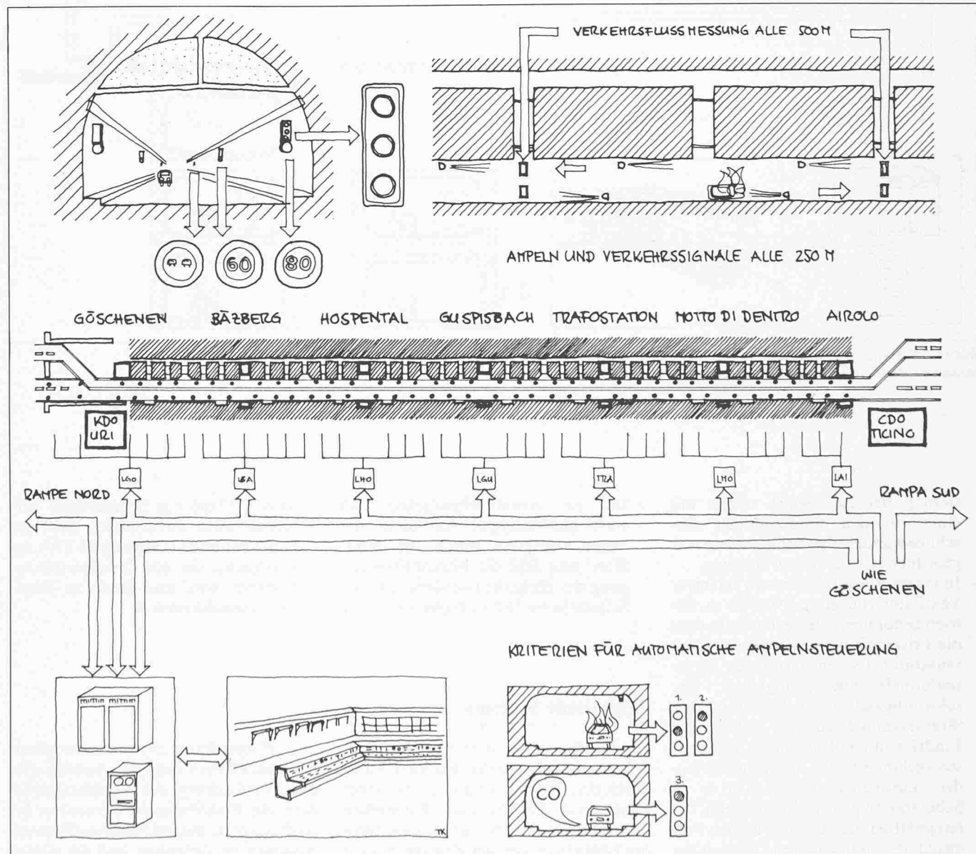
Bild 21. Verkehrssteuerung (schematisch)
