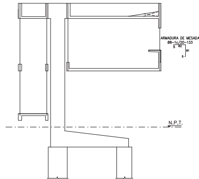
VISTA BB' OBS: Verificar medidas con planos de arquitectura
