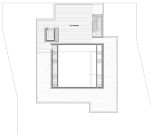
Grundriss 4. OG.
