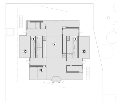
Grundriss EG.
