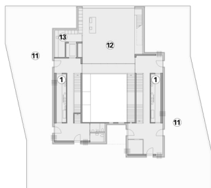
Grundriss 3. OG.
