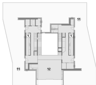
Grundriss 2. OG.
