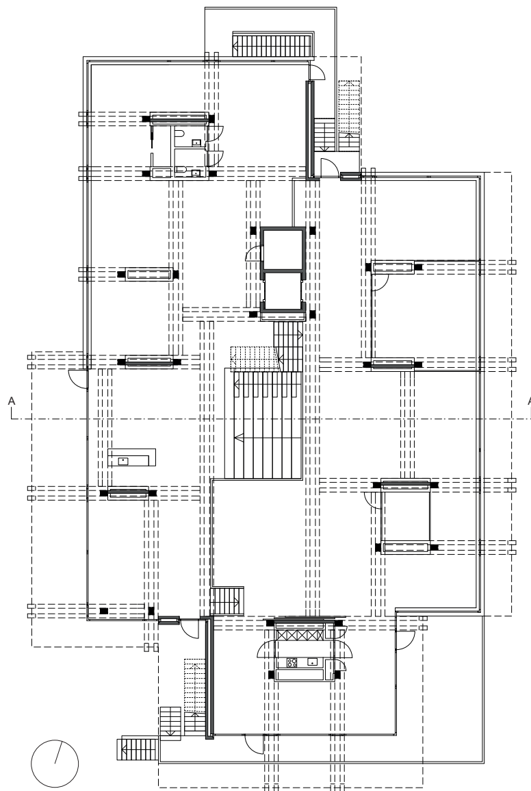
Grundriss Gartengeschoß
