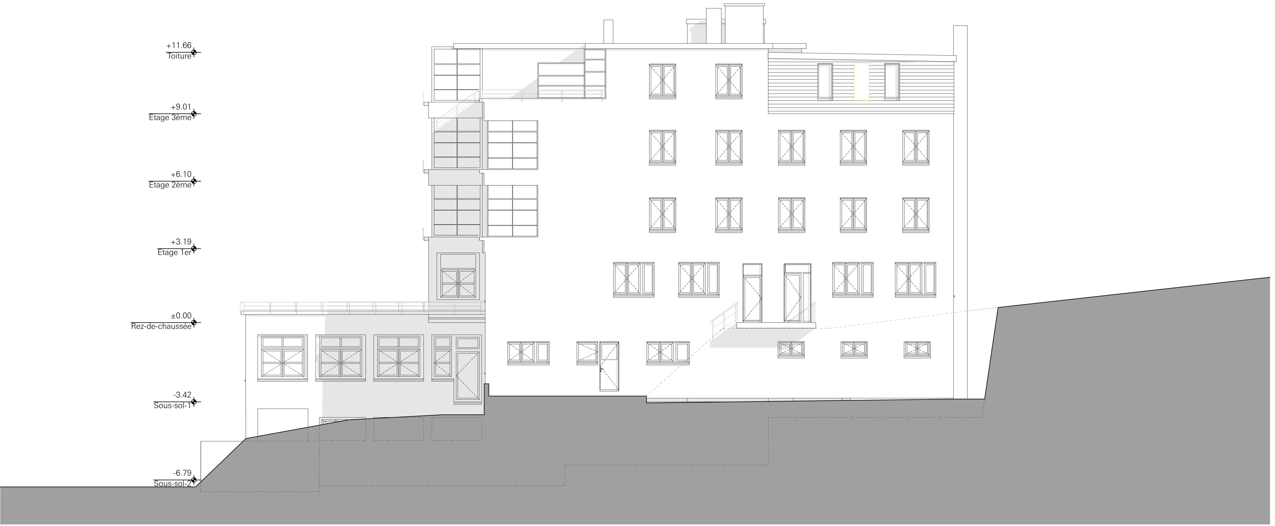
FACADE EST
