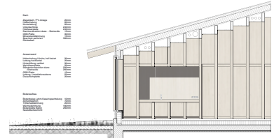
Korridorquerschnitt | 1:20
