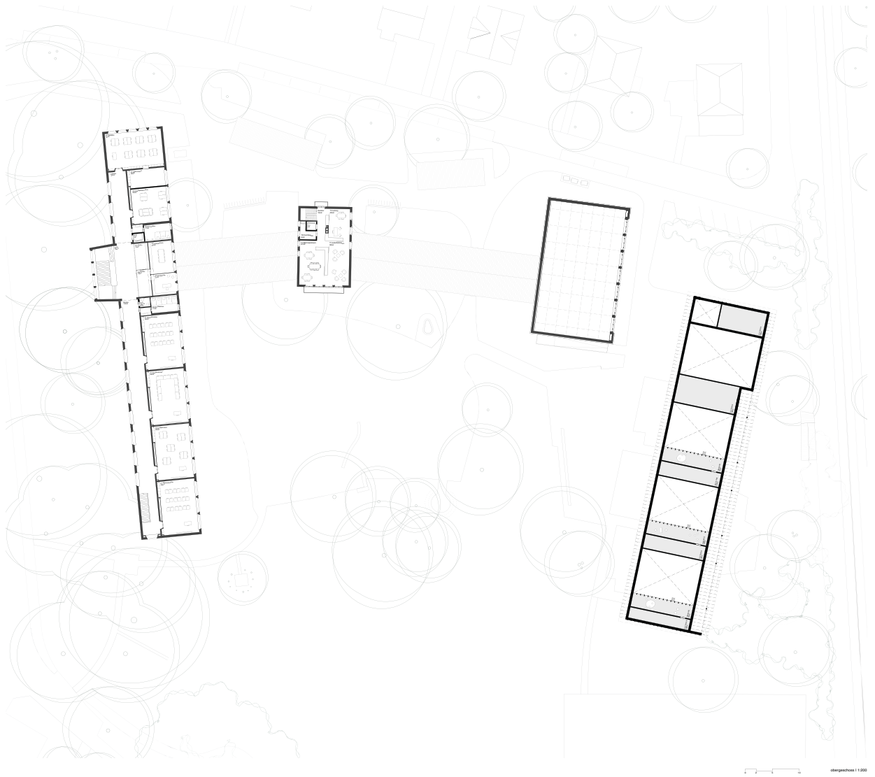
Übergangsbereich 1:200
