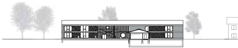
Längsschnitt G-G M 1:500
