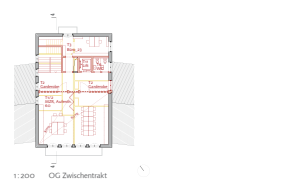
1:200 OG Zwischenstrakt
