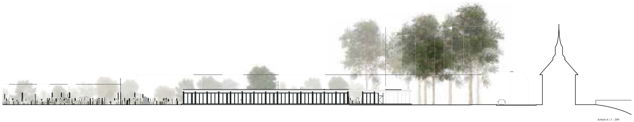
Schnitt A / 1 : 200
