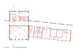
1:200 EG Zwischenstrakt
