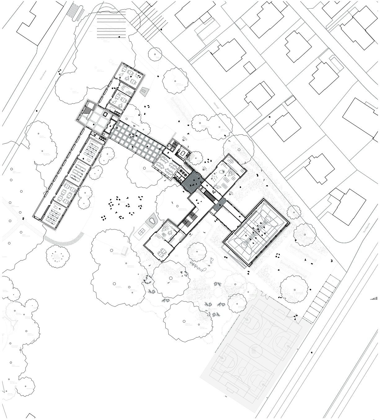
Erdgeschoss M 1:500
