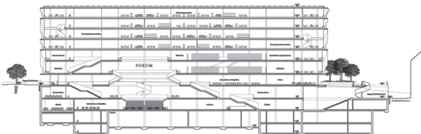
Schnitt Nord-Süd 1:800
