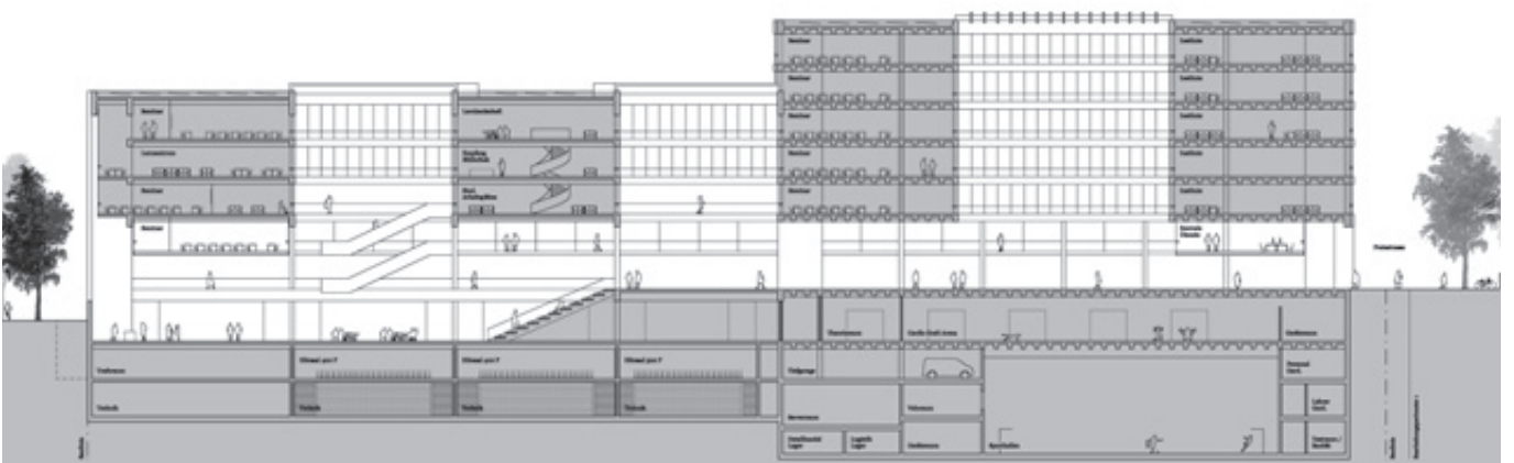
Schnitt West-Ost 1:800
