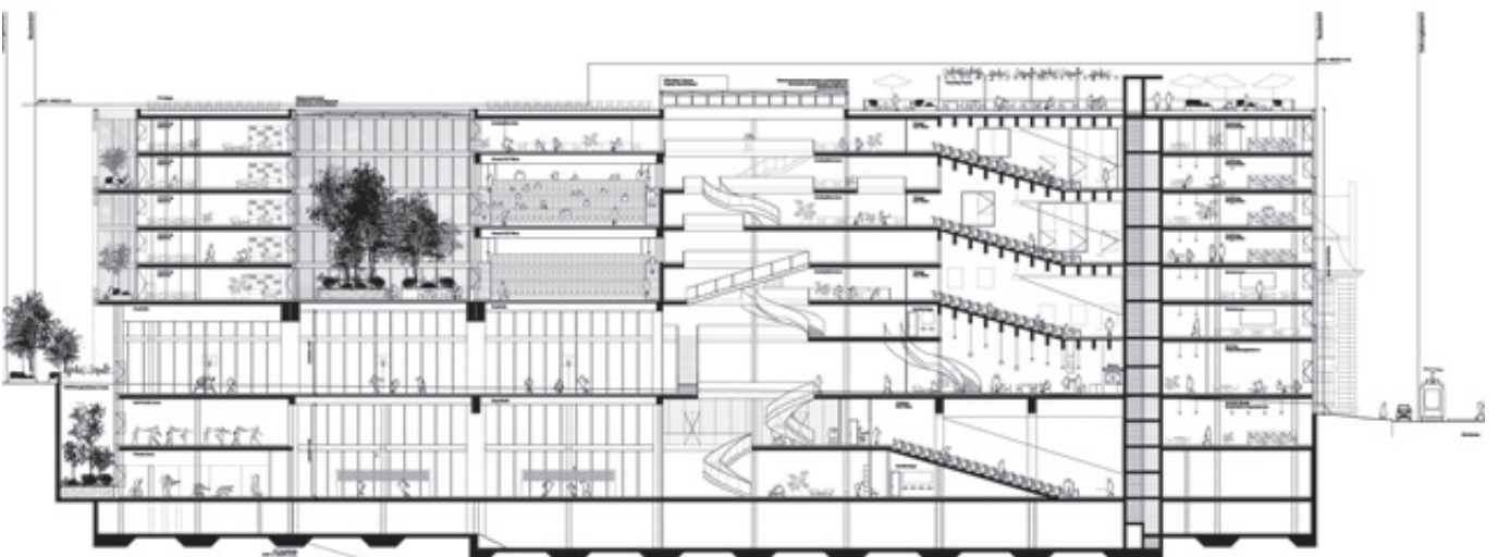
Längsschnitt Ost-West 1:800
