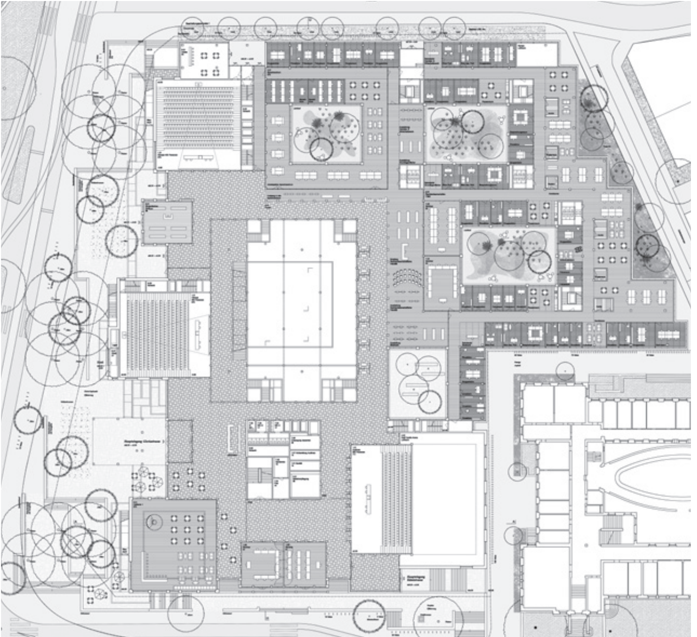
Erdgeschoss 1:850
