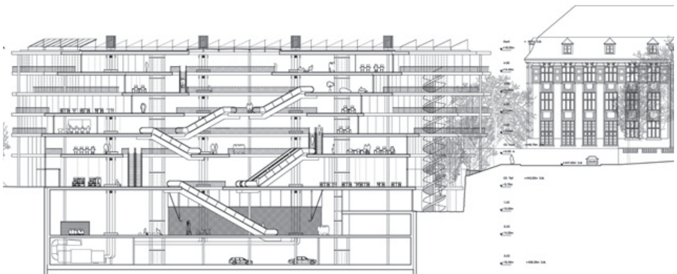
Querschnitt Süd-Nord 1:800
