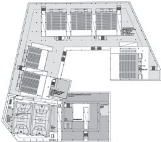
3. Obergeschoss 1:2000
