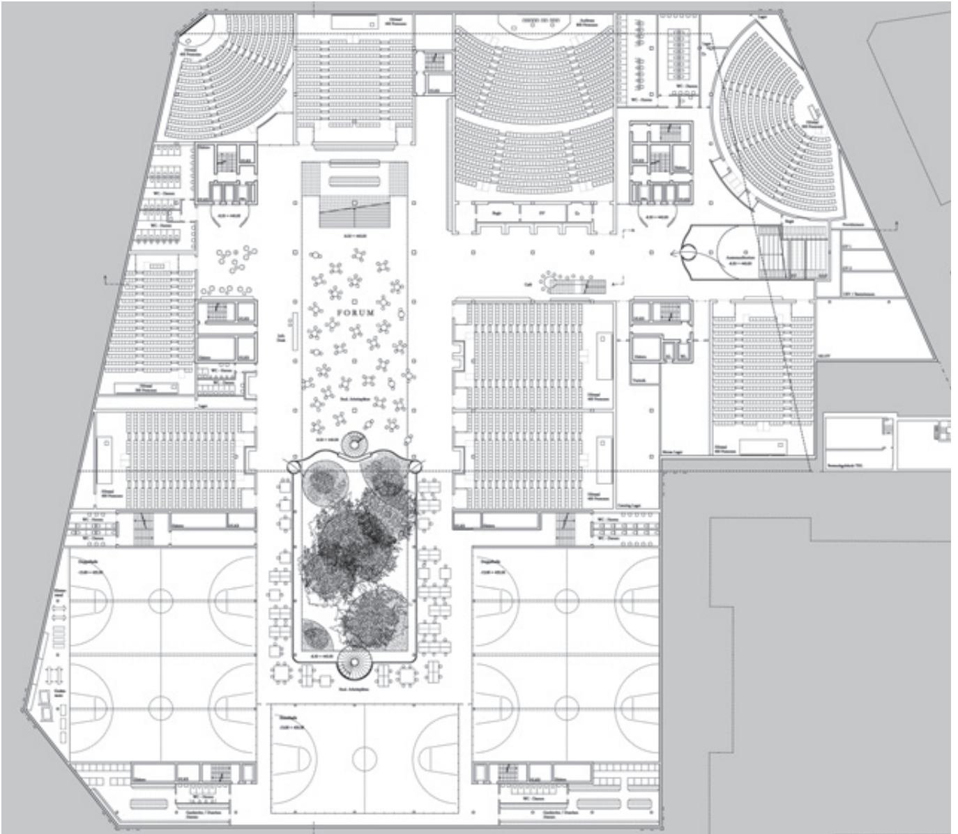
2. Untergeschoss 1:800
