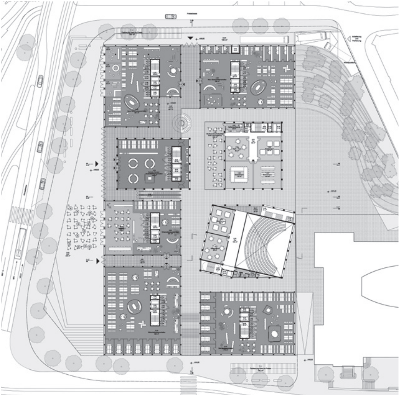
Platzebene 1:850
