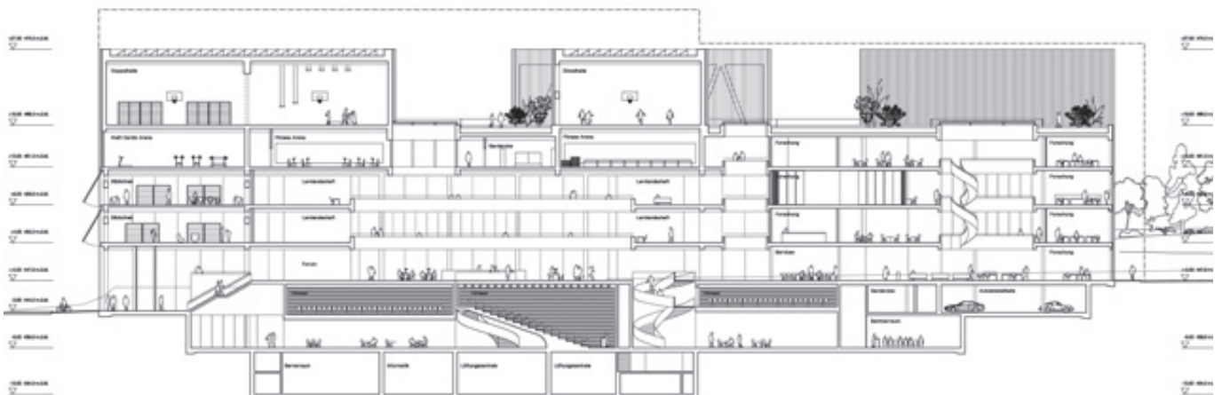
Schnitt West-Ost 1:800
