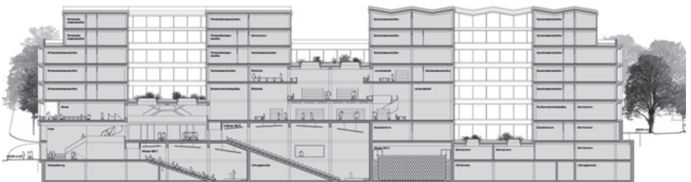
Schnitt West-Ost 1:800
