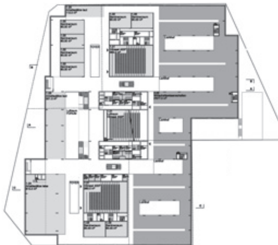
2. Obergeschoss 1:2000
