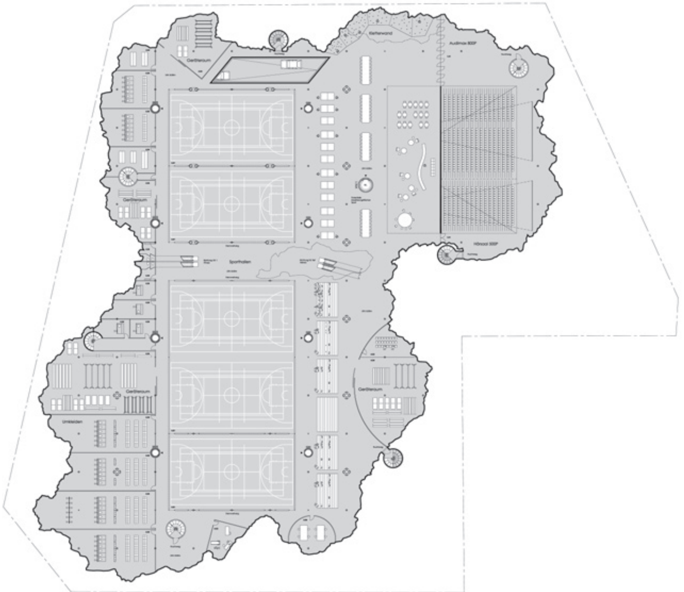
2. Untergeschoss 1:800
