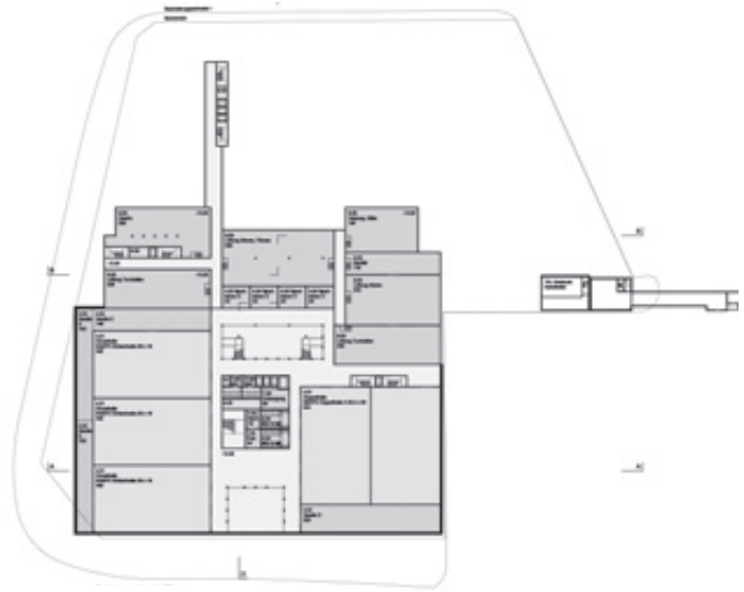
3. Untergeschoss 1:2000
