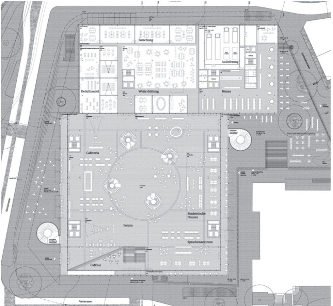
Erdgeschoss 1:850
