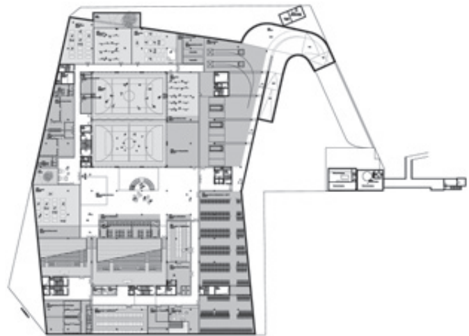
Untergeschoss 1:2000
