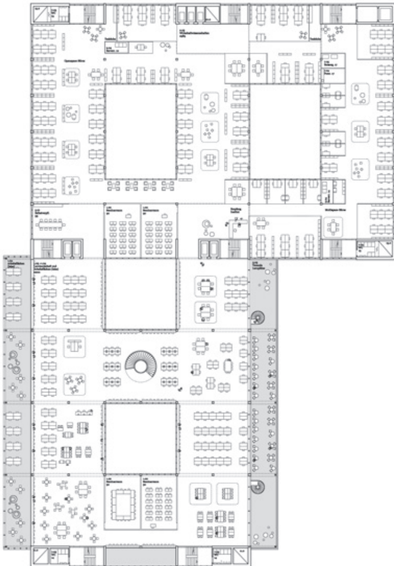
3. Obergeschoss 1:800
