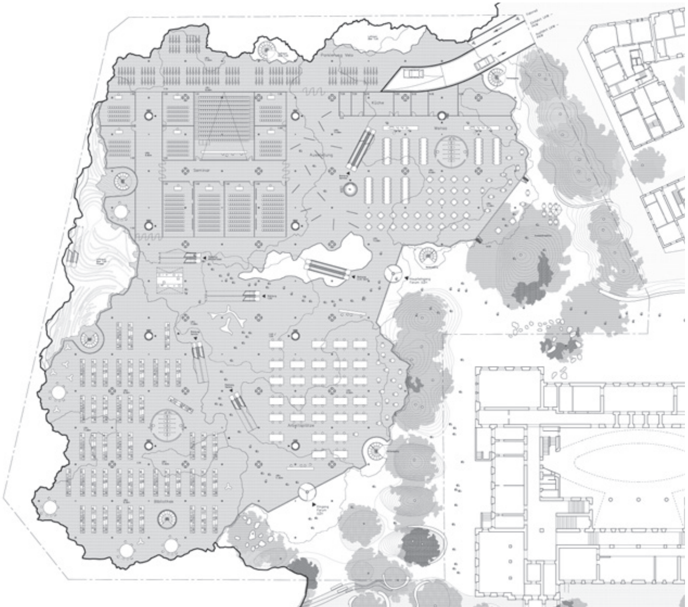
Erdgeschoss tief 1:850
