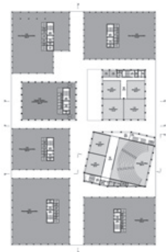
1. Obergeschoss 1:2000
