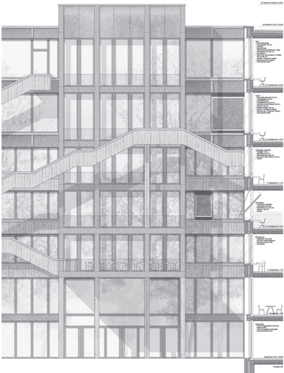
Konstruktionsschnitt mit Ansicht 1:150
