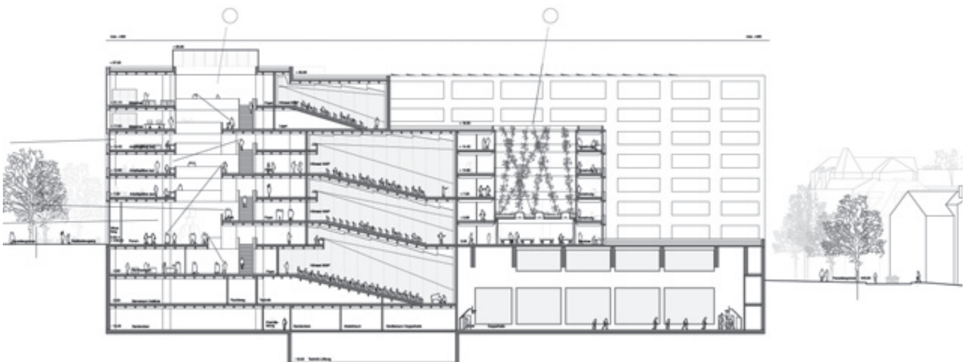
Schnitt Nord-Süd 1:800
