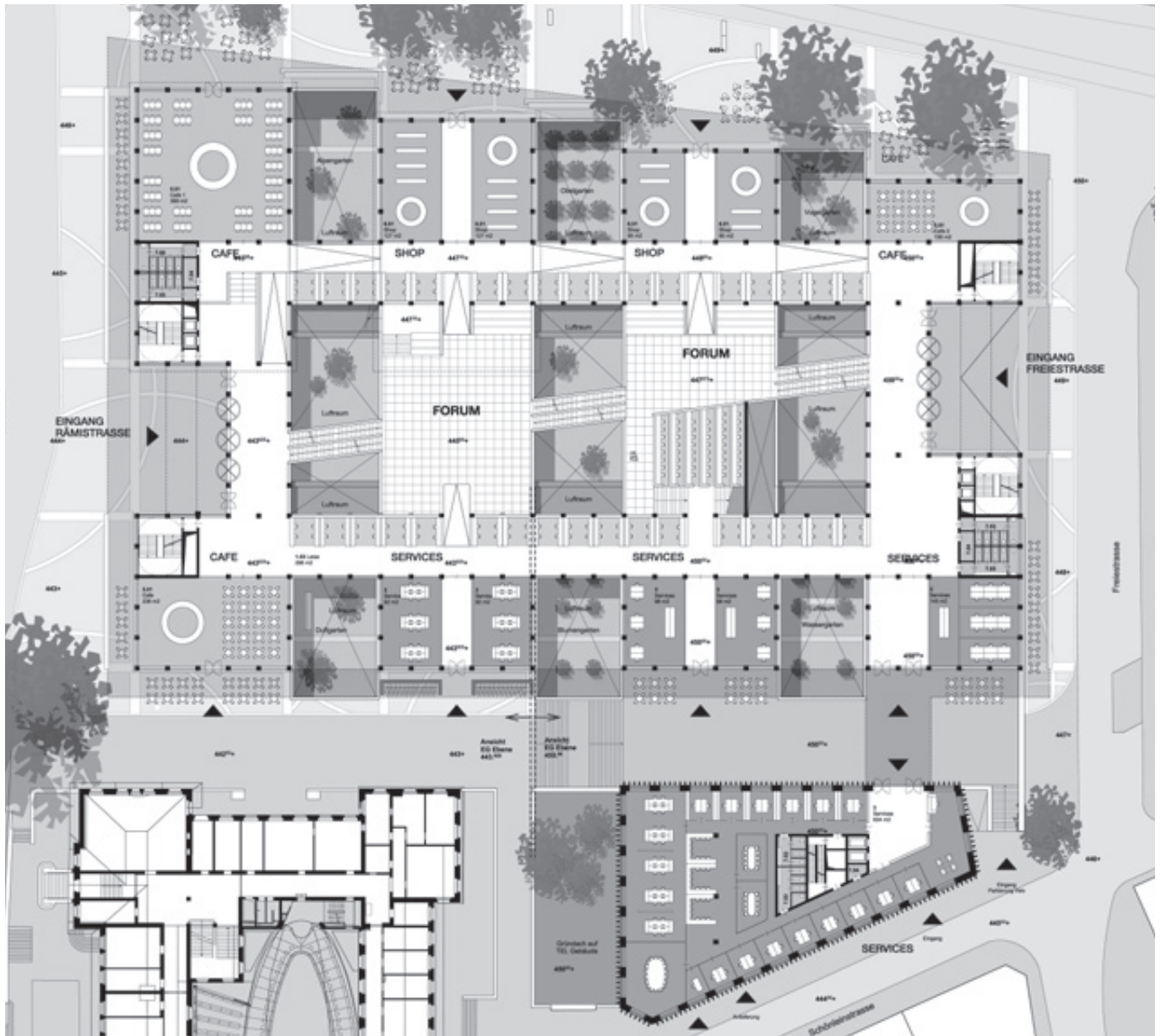
Erdgeschoss Rämistrasse/Gloriastrasse/Freiestrasse 1:850
