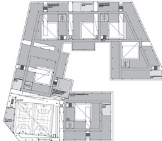
5. Obergeschoss 1:2000
