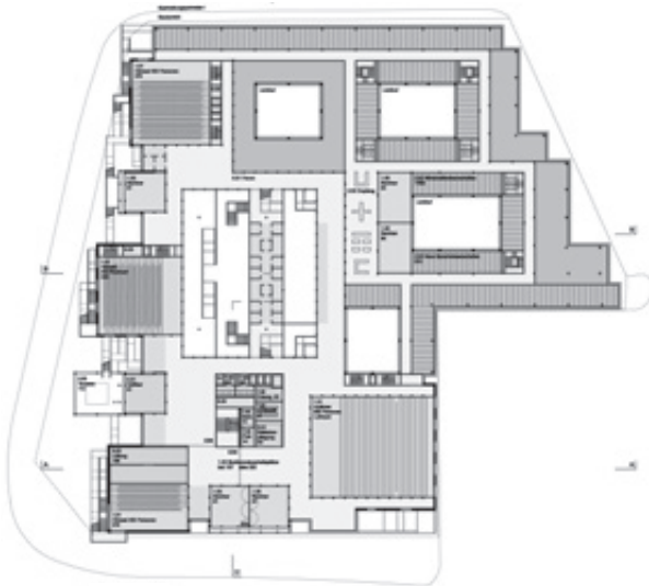
2. Obergeschoss 1:2000
