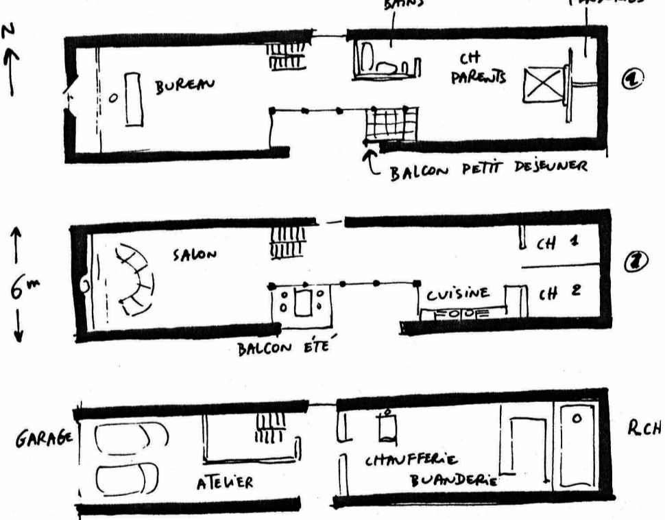
PLAN DES TROIS ÉTAGES - AUCUNE PORTE - FA ÇÔTÉ CHER ET C'EST INUTILE SI LE PLAN EST BIEN FAIT!
