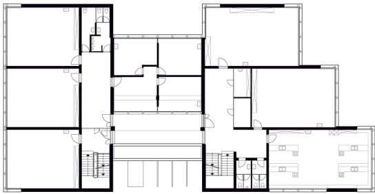
Grundriss 1. OG vor dem Umbau
