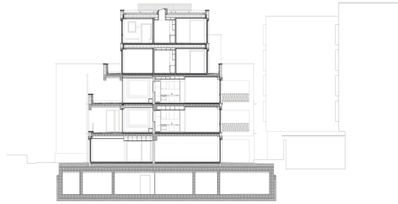
Querschnitt neu
