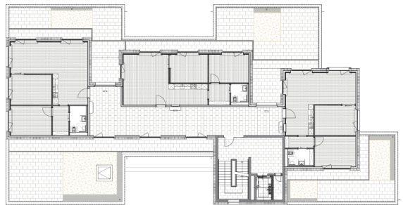
Grundriss 3. OG neu
