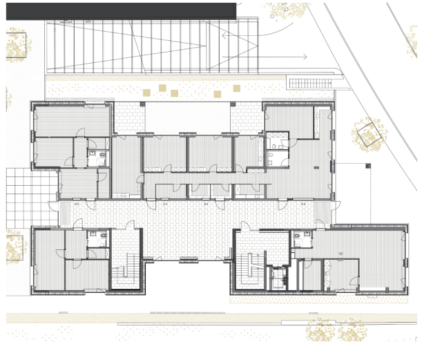
Grundriss EG neu
