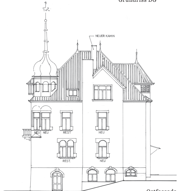
Ostfassade
