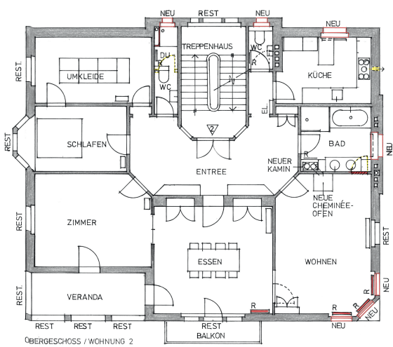
ÜBERGESCHOSS / WOHNUNG 2
