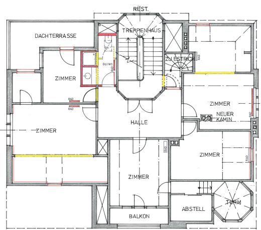
Grundriss DG
