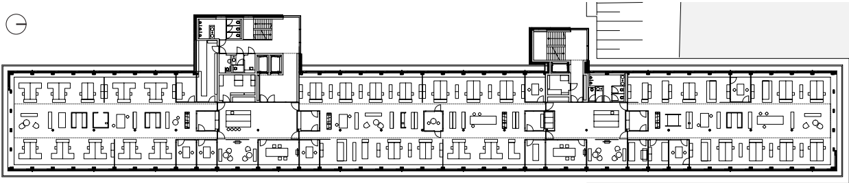
Die Bürogeschosse werden durch die Treppenhäuser und ihnen angeschlossene Aufenthaltsräume in drei Teile gegliedert. Regelgrundriss Arbeitsgeschoss
