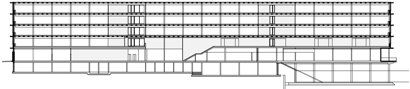
Längsschnitt: Im Schnitt ist der betonierte Sockel ersichtlich, auf dem der Holzbau steht.
