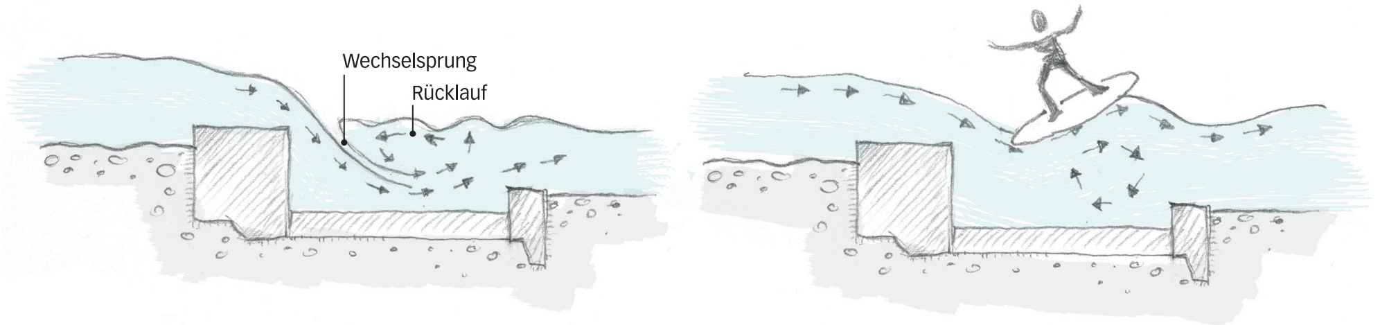
Wasserbaulich optimierte Energieumwandlung (links) und stehende Welle (rechts). 3
