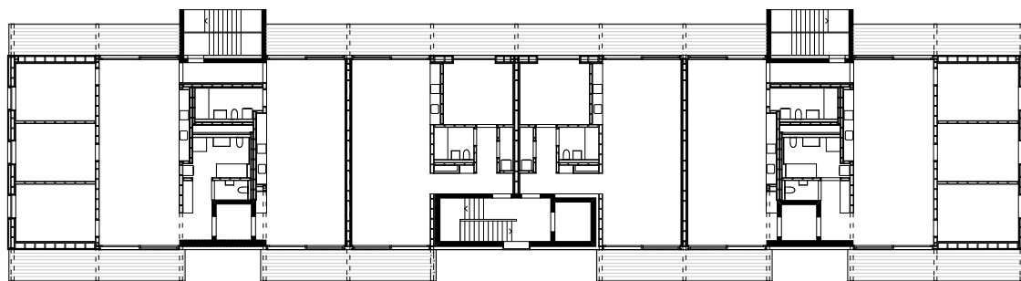
Grundriss Aufstockung.
