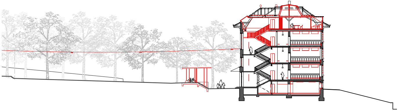
Schnitt Schulgebäude mit Pausenplatz, M 1:500
