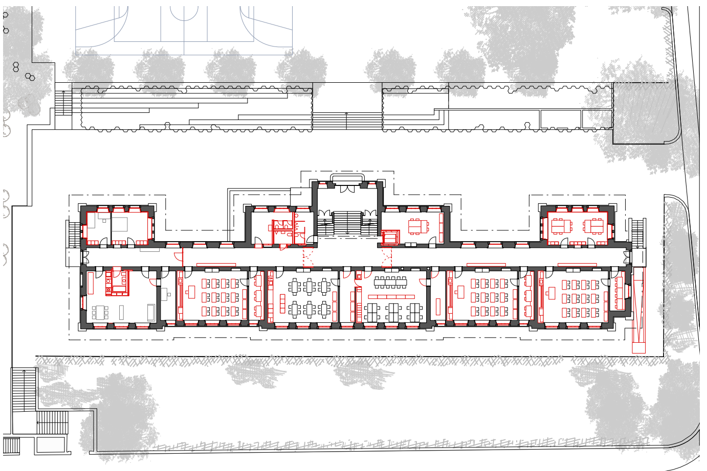
Erdgeschoss mit Umgebung, M 1:500
