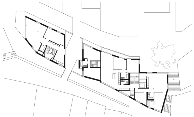
Pianta livello 3
