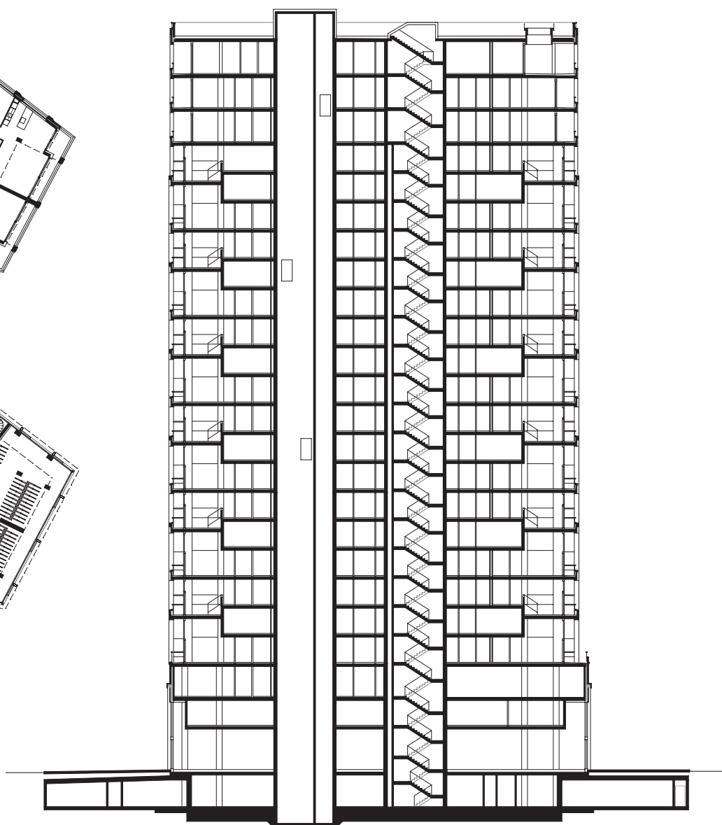
Sezione
