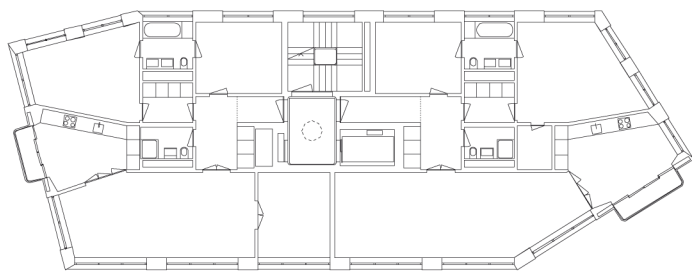
Pianta livelli 1-4
