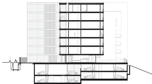
Sezione trasversale
