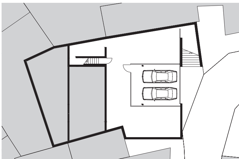
Pianta piano cantina
