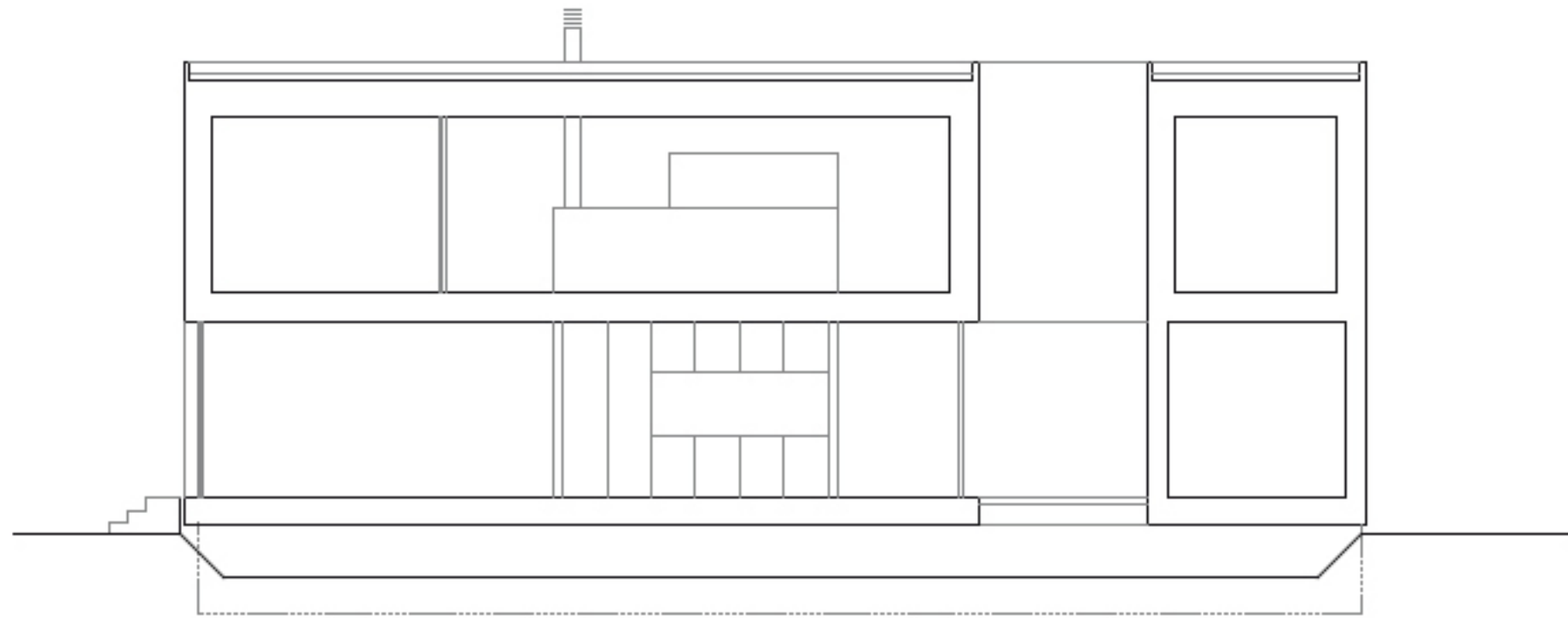
Sezione longitudinale
