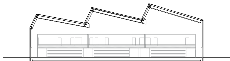
Sezione longitudinale
