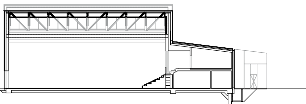
Sezione trasversale
