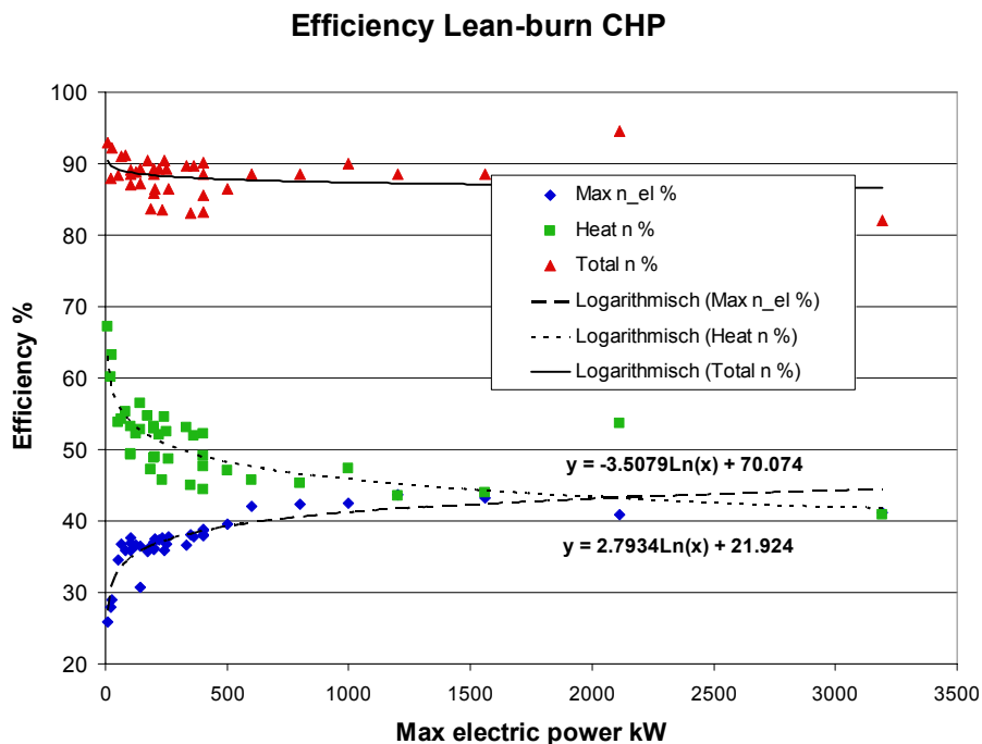
Abbildung 3 Wirkungsgrade der Magermotoren in Abhängigkeit von der Anlagenleistung und die zugehörigen Näherungskurven, ermittelt anhand von Herstellerangaben. 15 Rot: Gesamtwirkungsgrade; blau: elektrische Wirkungsgrade; grün: thermische Wirkungsgrade. „CHP“: „Combined Heat and Power“.
